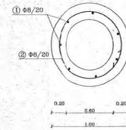
ΟΠΛΙΣΜΟΣ ΛΑΙΜΟΥ ΦΡΕΑΤΙΟΥ
