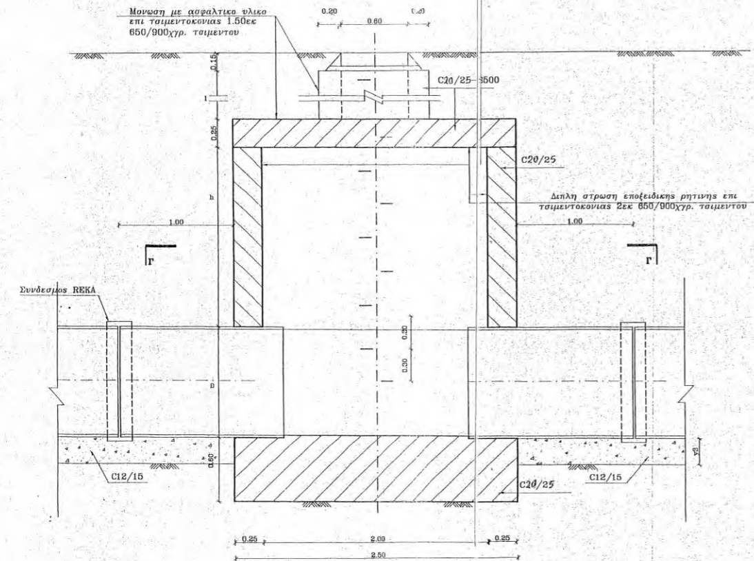
ΤΟΜΗ Α-Α
